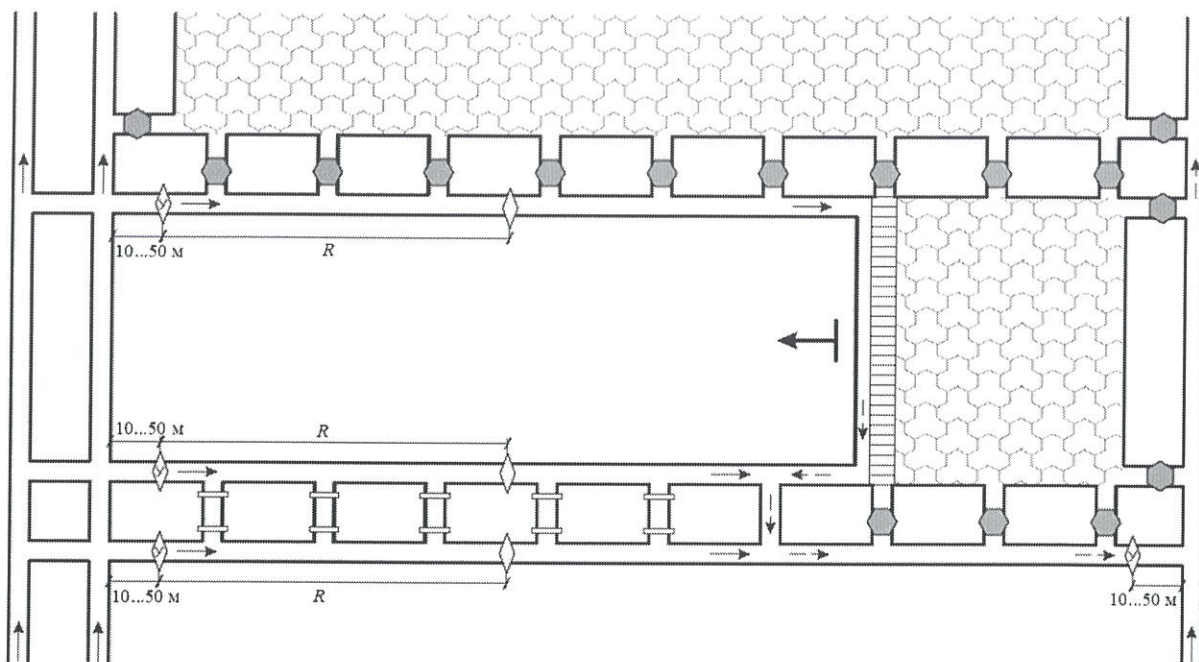
Рисунок 3 – Схема установки средств ВЗГВ для выемочного участка с возвратноточной схемой проветривания, подготовленного спаренными выработками
