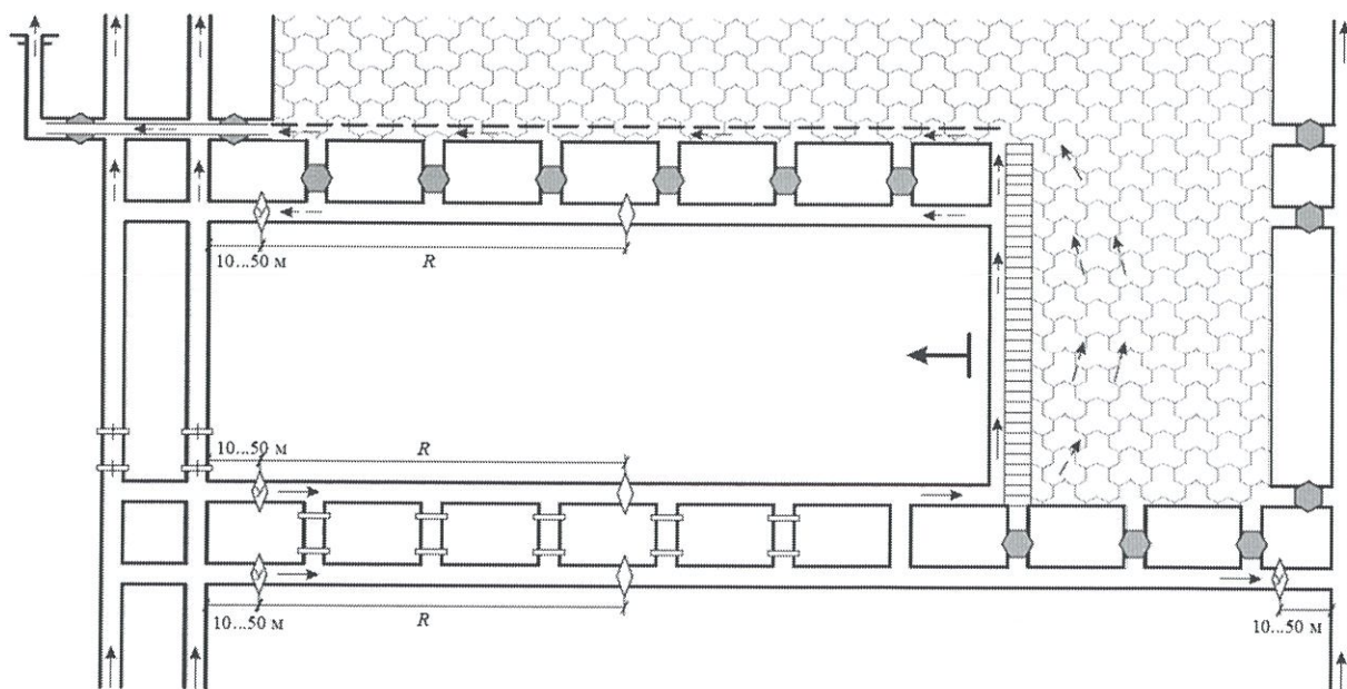
Рисунок 6 – Схема установки средств ВЗГВ для выемочного участка при проветривании с изолированным отводом метановоздушной смеси через выработанное пространство действующего и ранее отработанного выемочного столба
