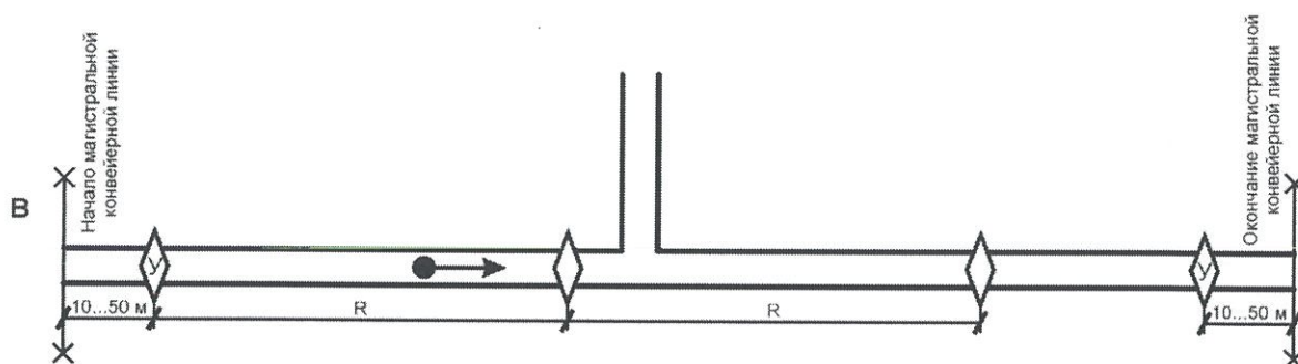
Рисунок 8 – Схема установки средств ВЗГВ для магистральных выработок, оборудованных ленточными конвейерами,
