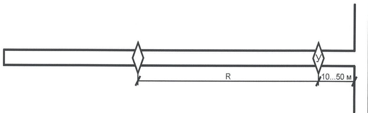
Рисунок 1 – Схемы установки средств ВЗГВ в подготовительной выработке
