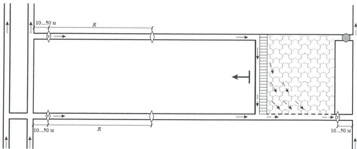
Рисунок 4 – Схема установки средств ВЗГВ для выемочного участка с прямой схемой проветривания
