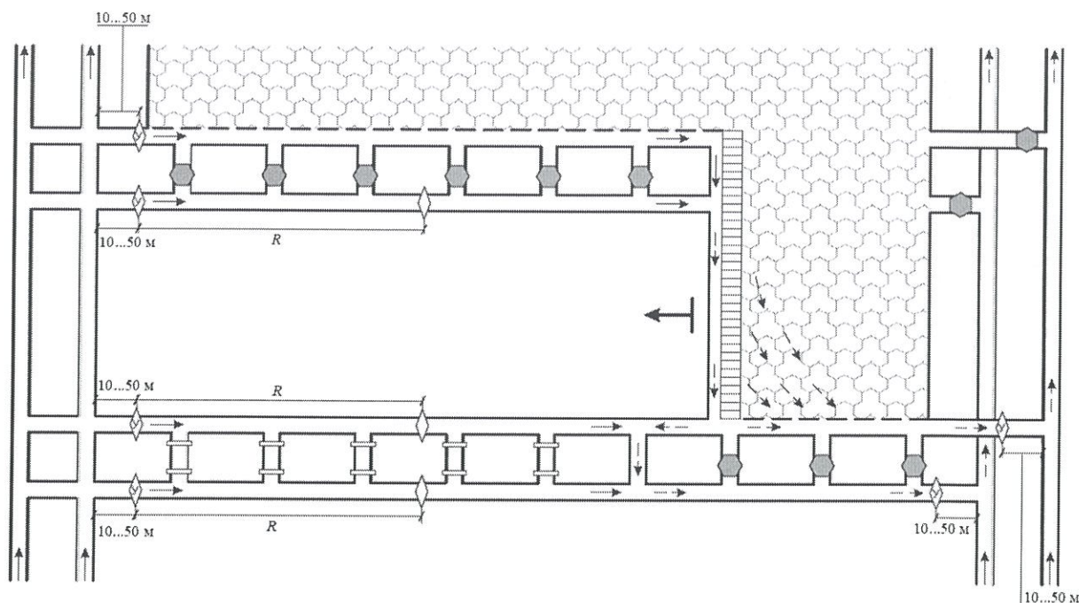
Рисунок 7 – Схема установки средств ВЗГВ для выемочного участка при проветривании с изолированным отводом метановоздушной смеси через выработанное пространство и сохраняемую в выработанном пространстве выработку
