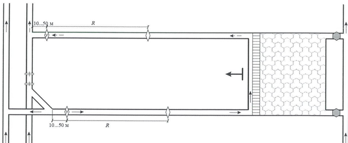
Рисунок 2 – Схема установки средств ВЗГВ для выемочного участка с возвратноточной схемой проветривания
